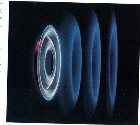
Normalt er det vanskeligt at kontrollere særligt de høje frekvensområder, hvis driverens areal er for stort. Det problem har Sennheiser snildt omgået ved at uforme membranen som en stor ring, i stedet for en stor skive.
